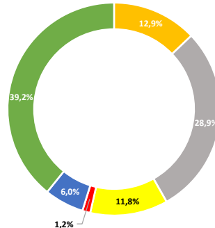
Durchschnitt Deutschland
