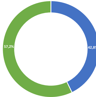
Siegtalstrom natur
