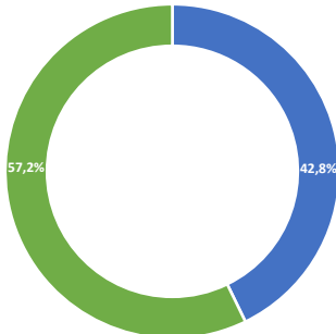
Verbleibender Energieträgermix
